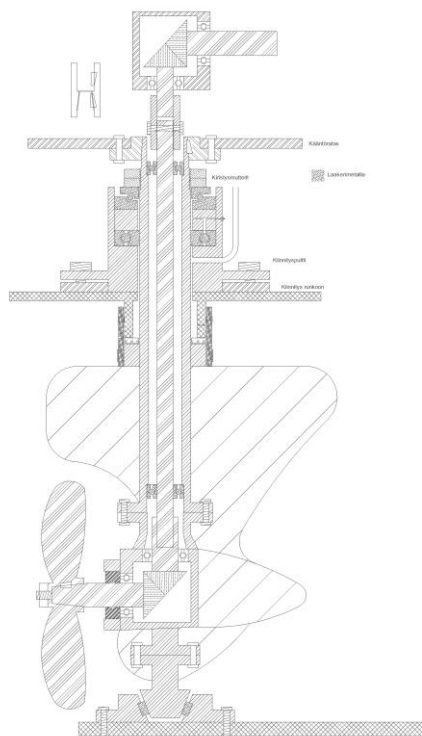
Kuva 7 vetolaitteen perusrakenne (Piirtänyt Eerik Ekström)
