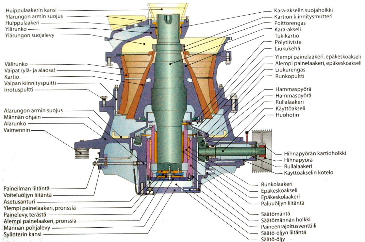
Kuva 2. GP-murskaimen poikkileikkaus. /3/
