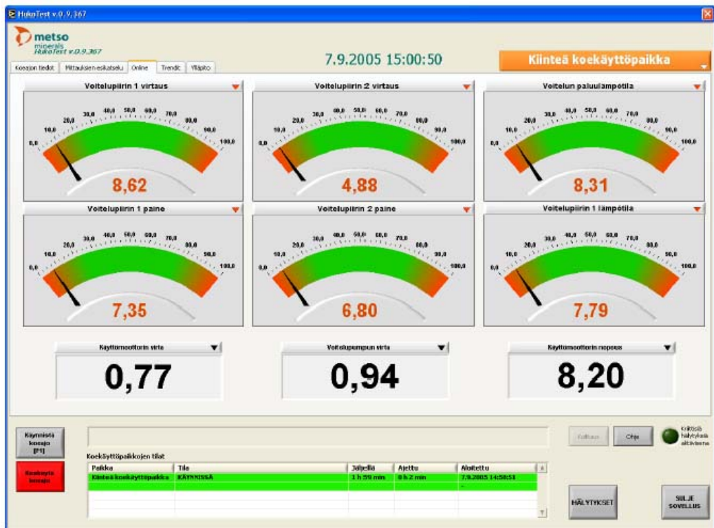
Kuva 8. Metso Mineralsin murskaimen koekäyttöjärjestelmän LabVIEW:lla toteutettu käyttöliittymä ja mittausten seuranta. /13/
