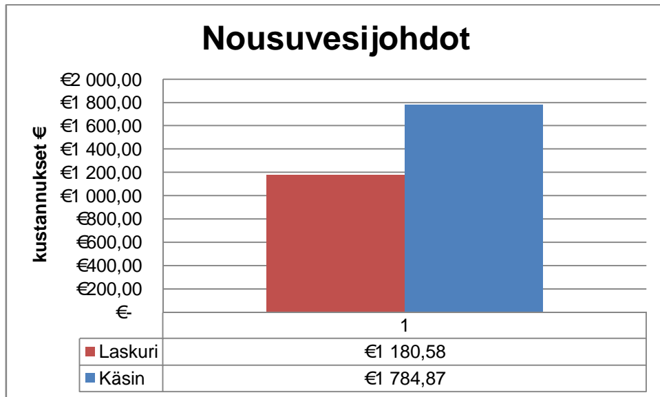
Kuva 11. Nousuvesijohtojen materiaalien hintaero
