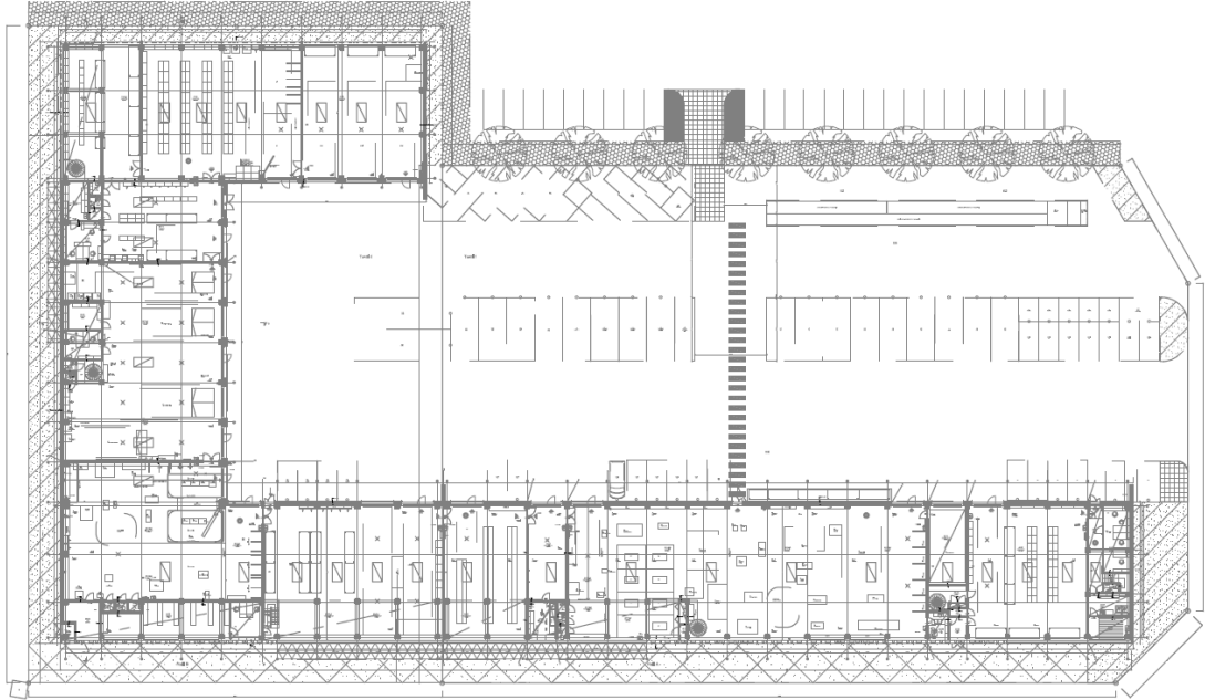
Kuva 14. Kerros 1. Vuosaaren tulevasta hallirakennuksesta. [11]
