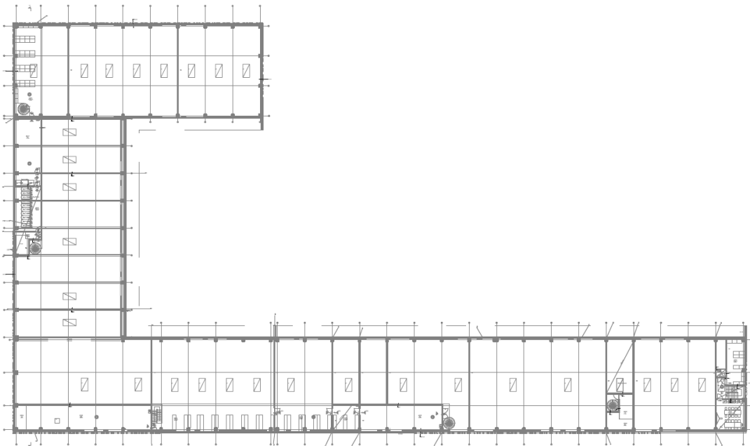
Kuva 15. Kerros 2. Vuosaaren tulevasta hallirakennuksesta. [11]
