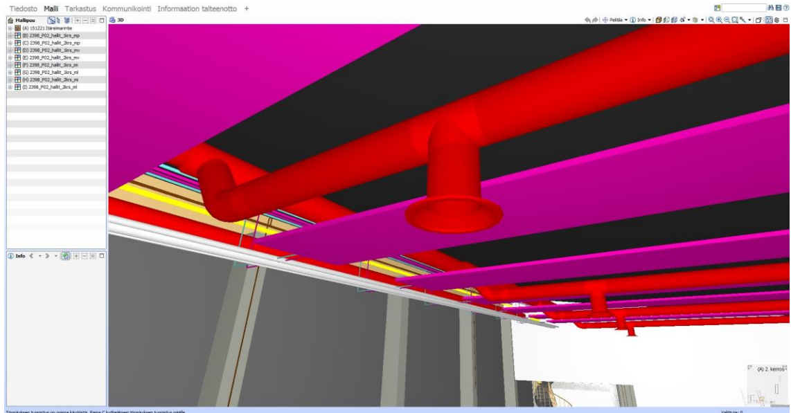
Kuva 11. Esimerkkikuva ilmanvaihtokanavistosta ja päätelaitteesta. [11]
