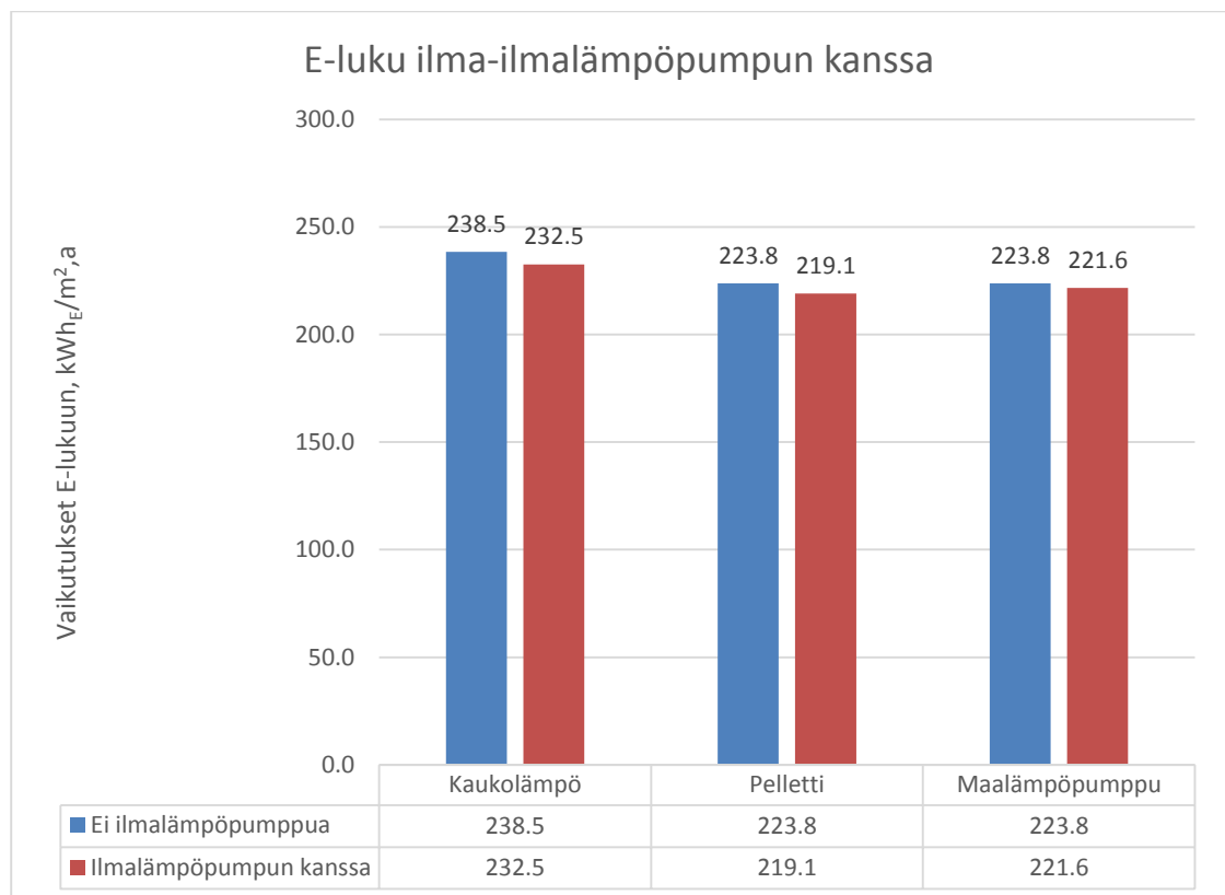
KUVA 16. E-luku ilma-ilmalämpöpumpun kanssa
