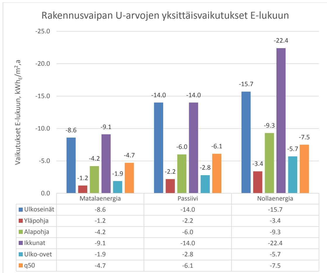
KUVA 9. Rakennusvaipan U-arvojen vaikutukset E-lukuun
