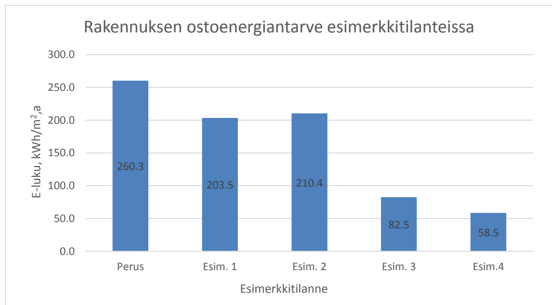
KUVA 17. Rakennuksen ostoenergiantarve esimerkkitalanteissa
