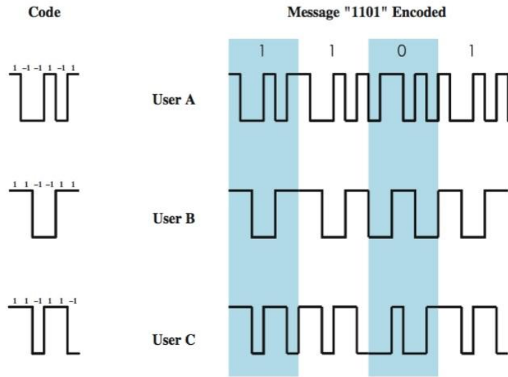
Kuva 14. Koodijakokanavointi
