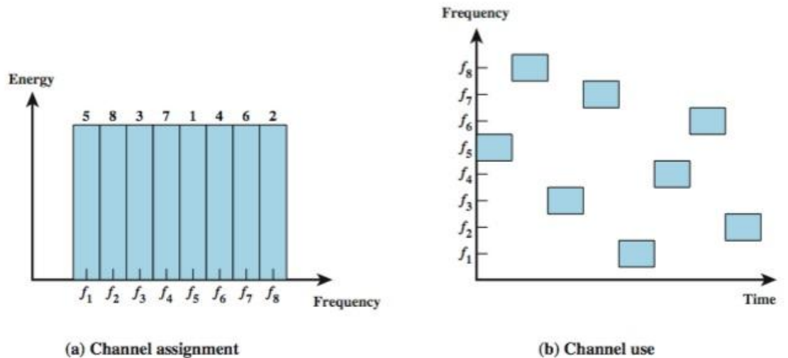
Kuva 7. Taajuushyppely [4.]
