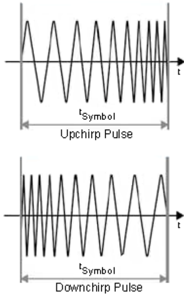
Kuva 10. Viserrysmodulaatio
