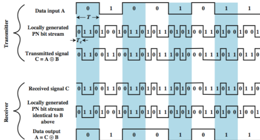
Kuva 8. Suorasekventointi. [4.]
