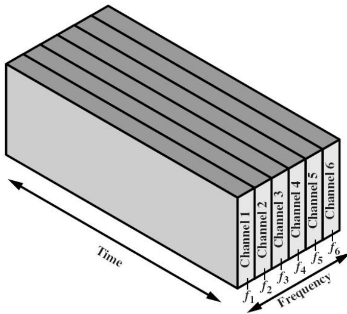
Kuva 11. Taajuusjakokanavointi [4.]
