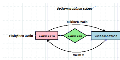
Kuva 8. Epäsymmetrinen salaus.
