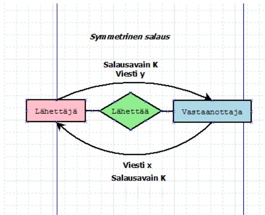
Kuva 9. Symmetrinen salaus.
