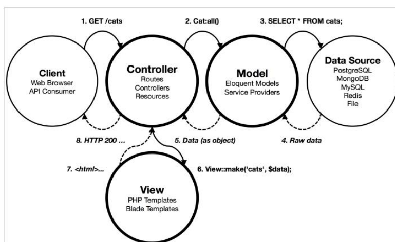
Kuva 3. HTTP-pyyntöä kulkeutuminen Laravelissa (6)
