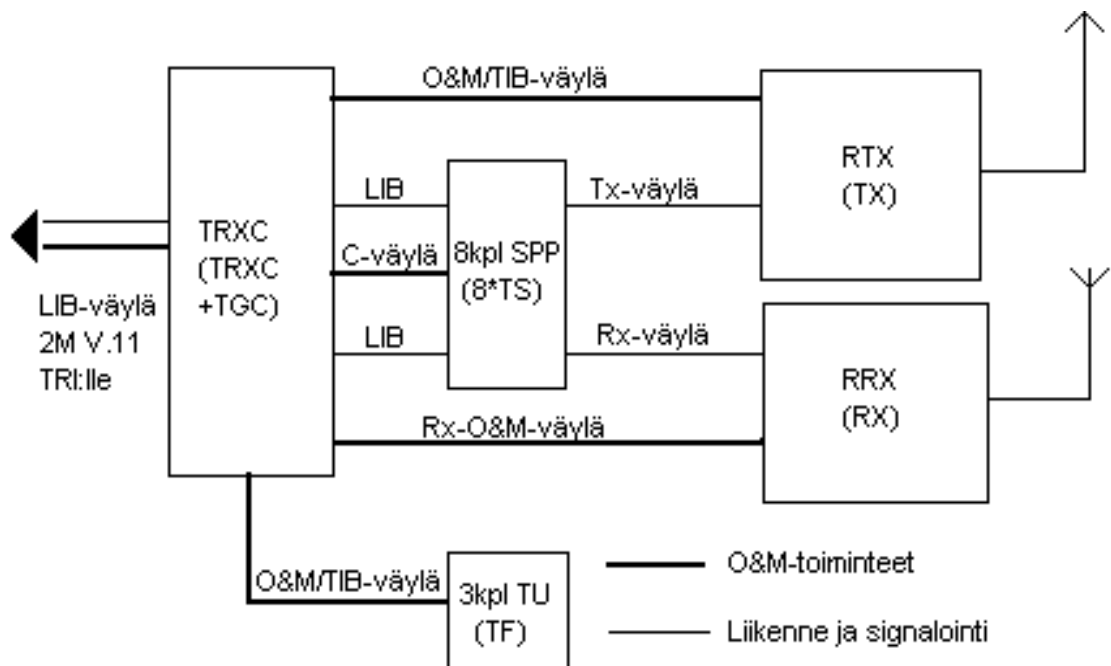
Kuva 4. TRX:n yksiköt ja väylöitykset [8]
