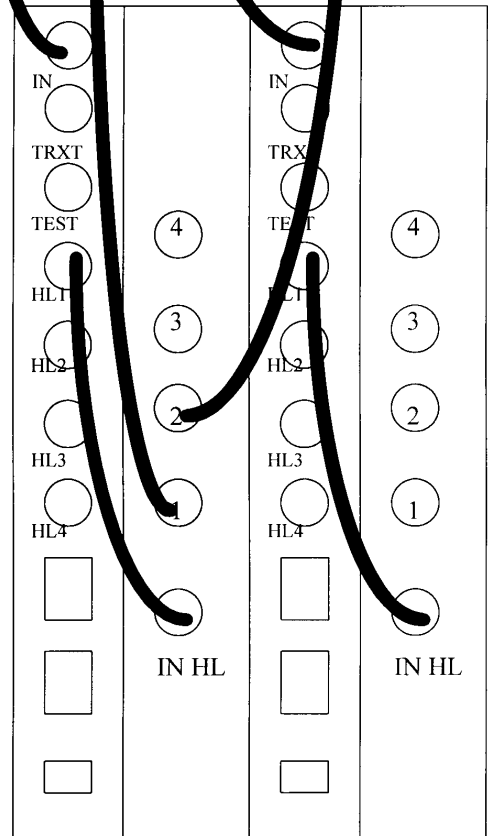
RX DIV MITTAUSKYTKENTÄ , PUHELUT OHJATTAVA MUIHIN SOLUIHIN MITATTAESSA
