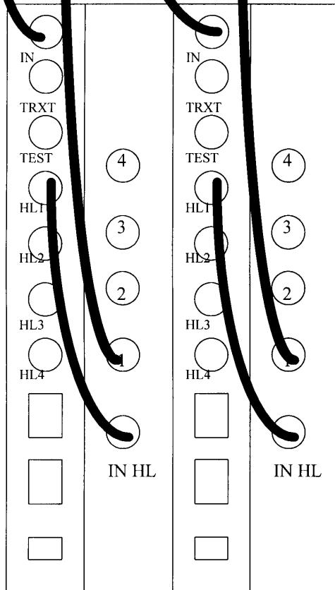
NORMAALI DIVERSITEETIKYTKENTÄ SEKÄ PSEUDO- ETTÄ NORMAALI DIVERSITEETTI
