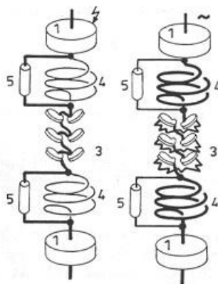
Kuva 12. Magneettipuhallussuojan rakenne. (1) Epälineaarinen vastus. (3) Aktiivikipinäväli. (4) Puhalluskäämit. (5) Puhalluskäämien ohitusvastukset. (Elovaara & Laiho 2007, 198; Aro ym. 2015, 344.)
