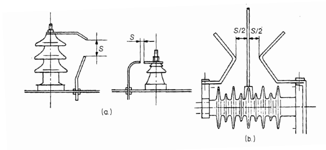
Kuva 9. Kipinävälirakenteet. (a) Yksivälisuoja. (b) Kaksivälisuoja. (Elovaara & Laiho 2007, 195)
