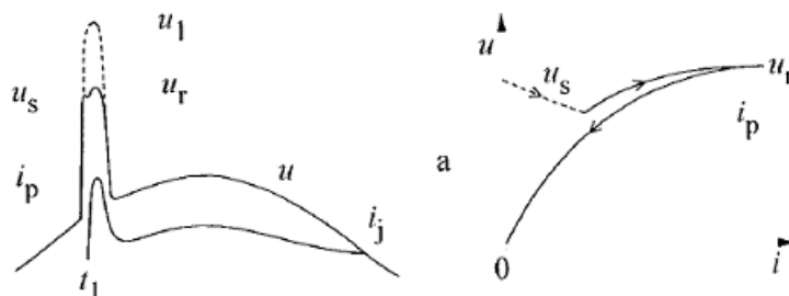
Kuva 11. Ylijännitteen rajoittuminen levykipinävälisuojan toimiessa ja suojan toimintapisteen siirtyminen. u_1 on tulevan ylijännitteen huippuarvo, u käyttötaajuinen jännitteen huippuarvo, u_s syttymisjännite, u_r jäänösjännitteen huippuarvo, i_p syöksyvirran huippuarvo, i_j jälkivirran huippuarvo ja t_1 syttymishetki. (Aro ym. 2015, 346.)
