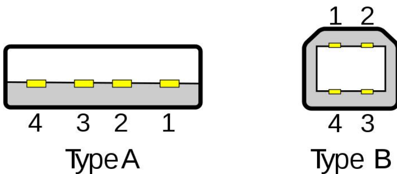
KUVA 5. USB-A ja USB-B -liittimet. Valkoiset alueet ovat tyhjiä (Duyé 2008)
