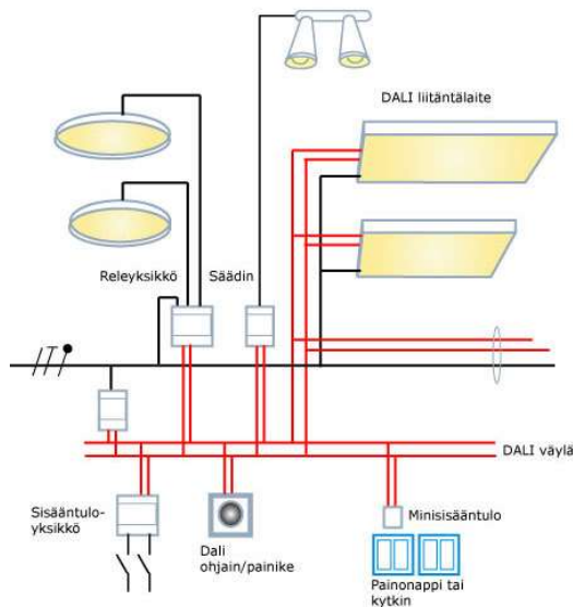
KUVA 4. DALI-väylän rakenne (5).
