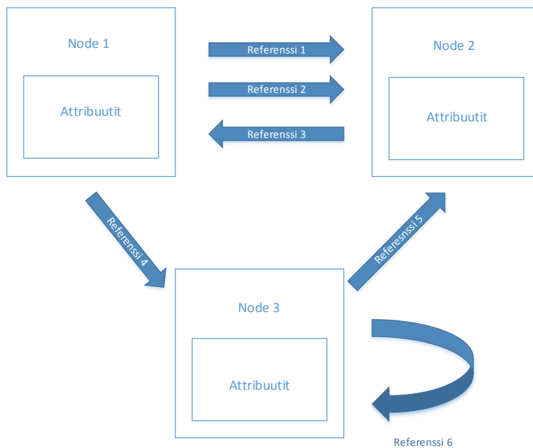
Kuva 6. OPC UA muodostuu yhtymäkohdista ja referensseistä, joilla on omat attribuuttinsa.
