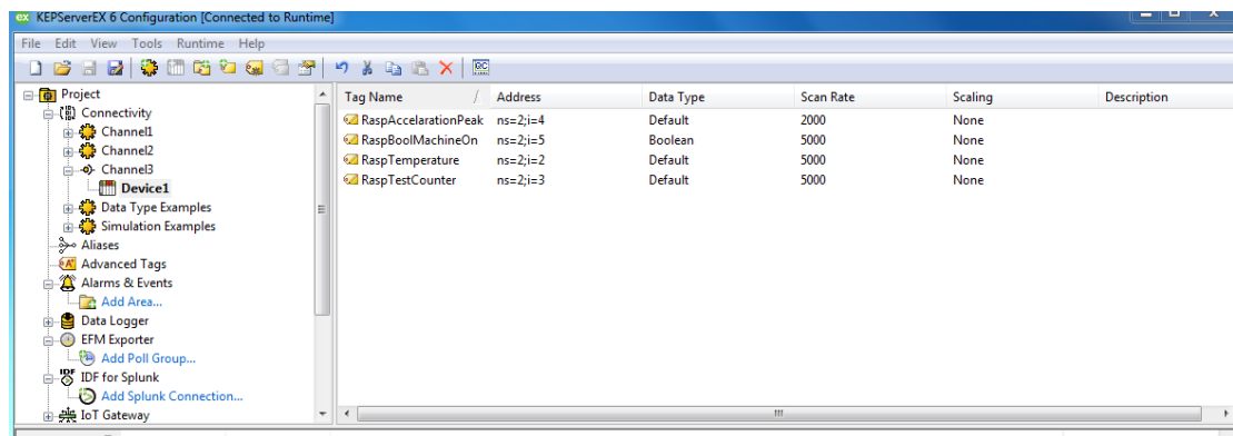
Kuva 20. KepwareServerEx 6 -ohjelmiston asetusnäkyä testimuuttujille
