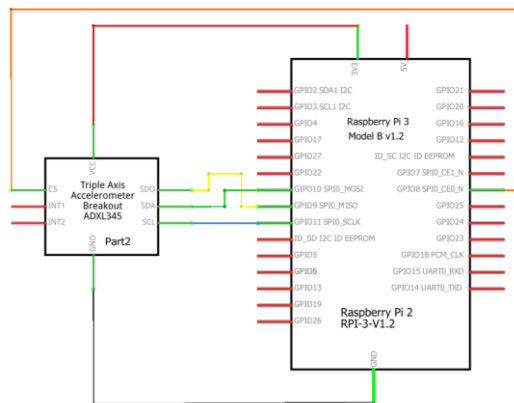
Kuva 18. Kytentäkaavio ADXL345-anturille Raspberry Pi -tietokoneeseen SPI-yhteyksikäytännöllä [35].
