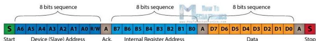
Kuva 10. I2C-yhteyshäytännö lähettää kolme 8 bitin sarjaa viesteissään [29].
