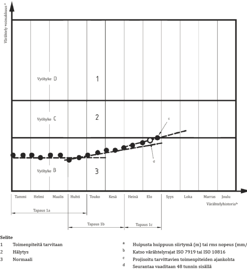
Kuva 3. Mitatun värähtelyn historiasta voidaan päätellä, milloin laitteen kunto alkaa heiketä ja milloin toimenpiteitä vaaditaan [5, s. 30].
