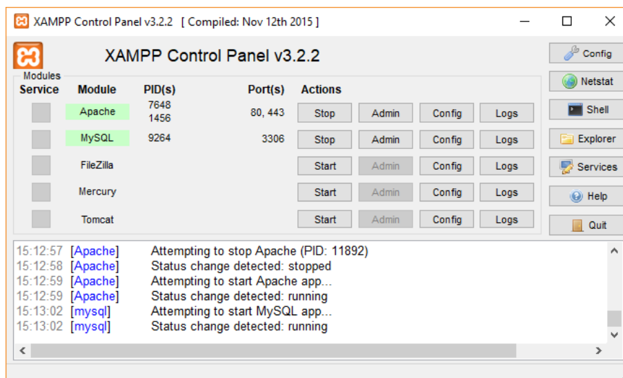
Figur 13. XAMPP kontrollpanel.
