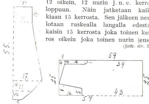
5. Pulloverin kaavat.
