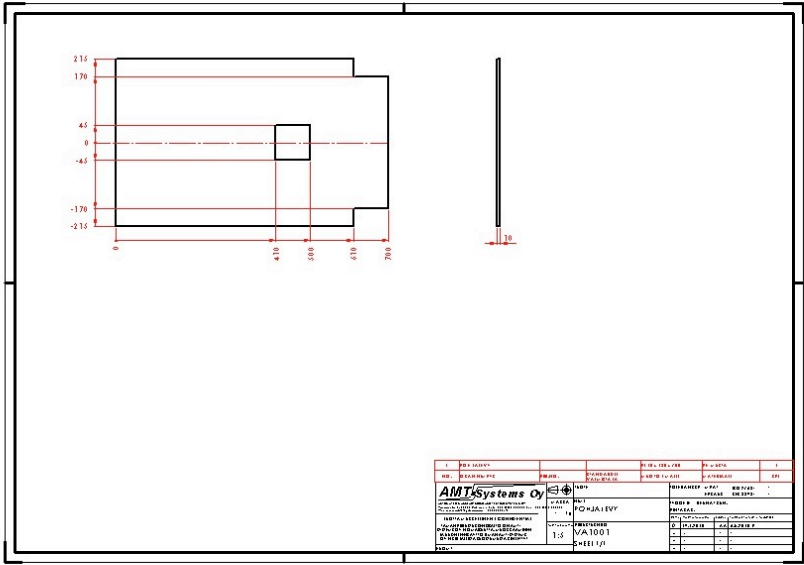
Liite 3: 2D-työpiirustus koordinaatistomitoituksella.
