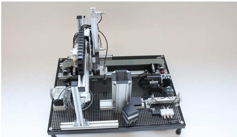
Kuva 9. LAI-harjoittelualusta, johon prototyyppi on tarkoitus asentaa jälkepäin (JJJ-Automaatio 2015).
