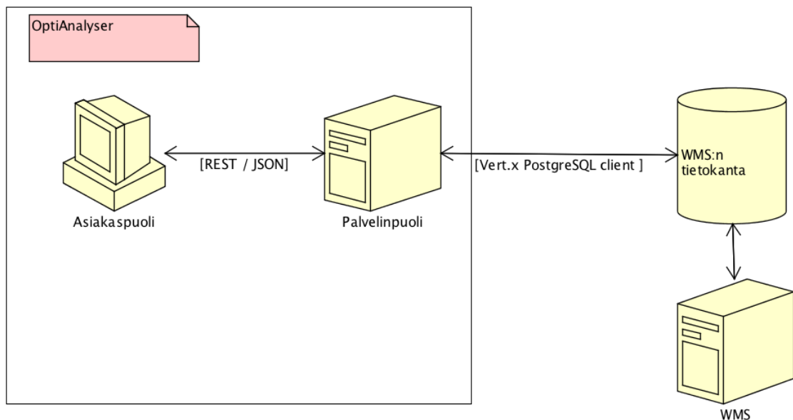
Kuva 10. OptiAnalyserin järjestelmäarkkitehtuuri
