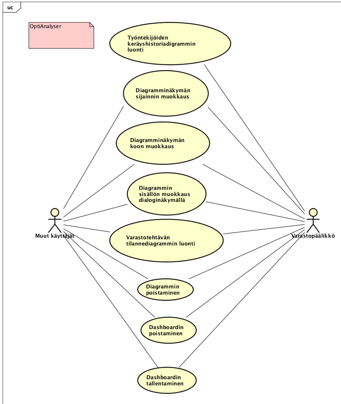
Kuva 9. OptiAnalyserin käyttötapaukset
