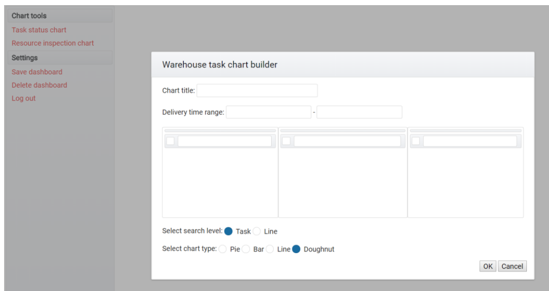
Kuva 17. Dialogikomponentin näkymä.
