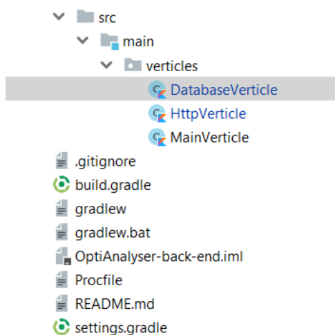
Kuva 19. Palvelinpuolen projektirakenne
