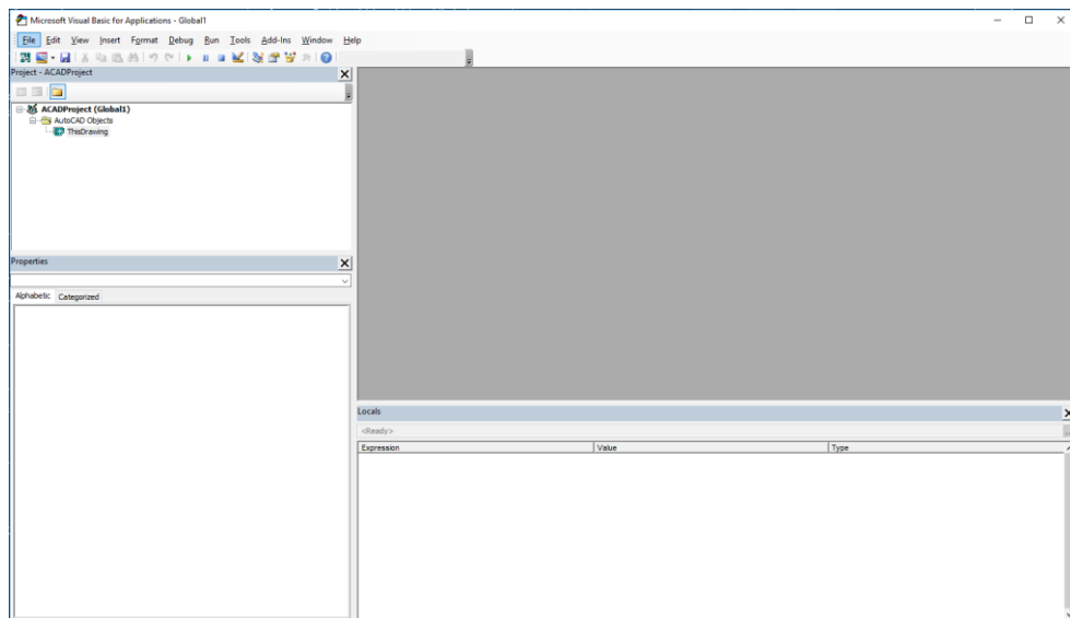
Kuva 7. Koodausympäristö
