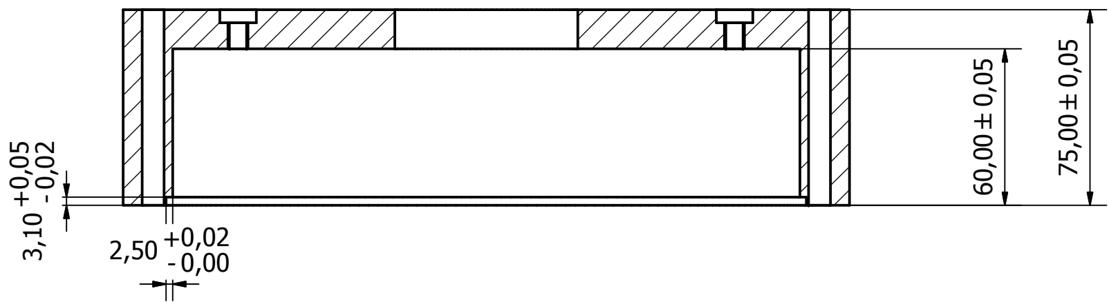
A-A ( 1 : 2 )
