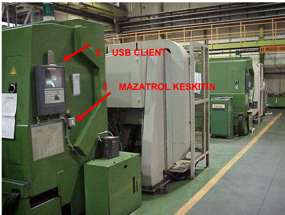
Kuva 3 USB Client ja keskitin NC-koneessa
