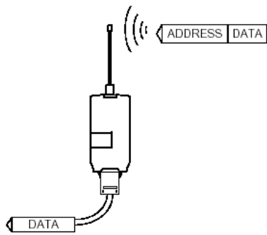
Kuva 7 Vastaanotto RX-osoitus päällä
