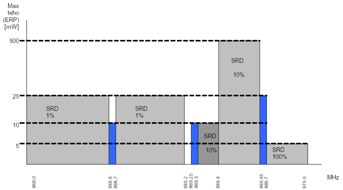
Kuva 4 Sallitut lähetystehot (ERP) ja toimitasuhteet (SRD) eri taajuuksilla (Lähde Satel Oy, ja viestintävirasto)
