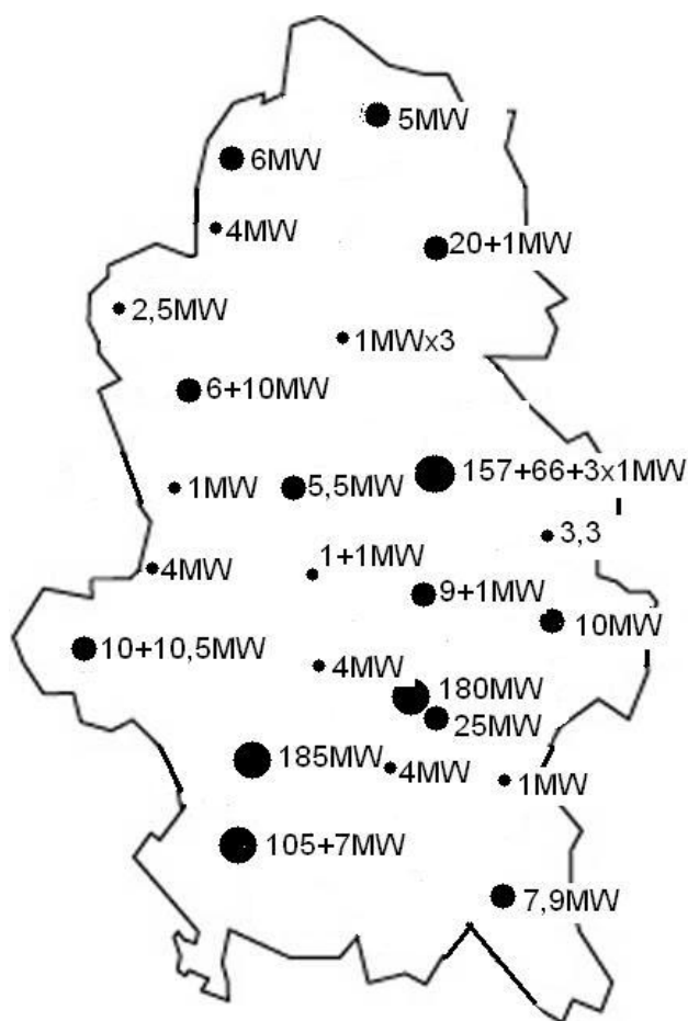
KUVIO 5. Voima- ja lämpölaitokset Keski-Suomessa > 1 MW
