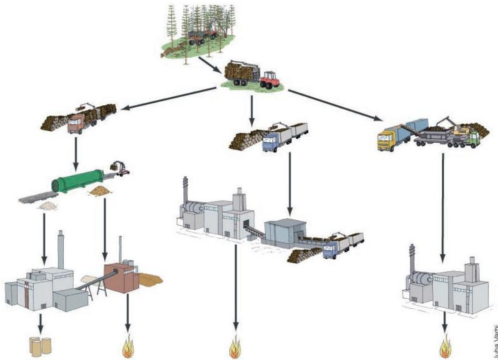
KUVIO 2. Kaaviokuva aines- ja energiapuun korjuuketjusta Fixteri-paalaimella (Biotukki Oy 2009)
