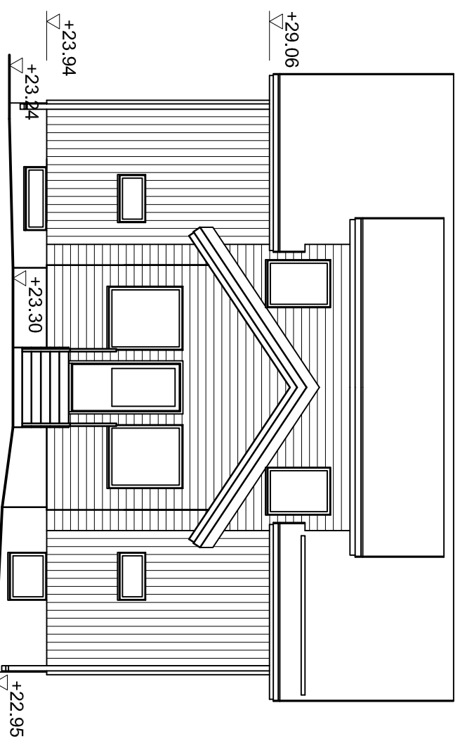
JULKISIVU KOILLISEEN
