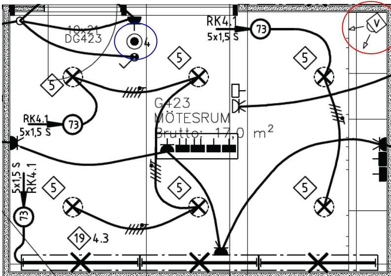
Figur 12 Elritning på mötesrum G423.
