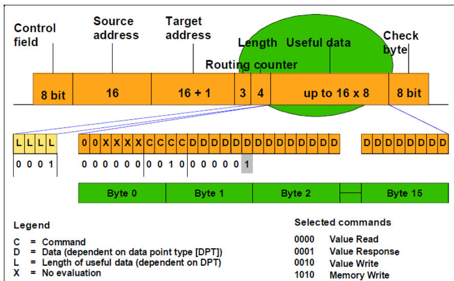
Figur 4 Telegrammens uppbyggnad /8/
