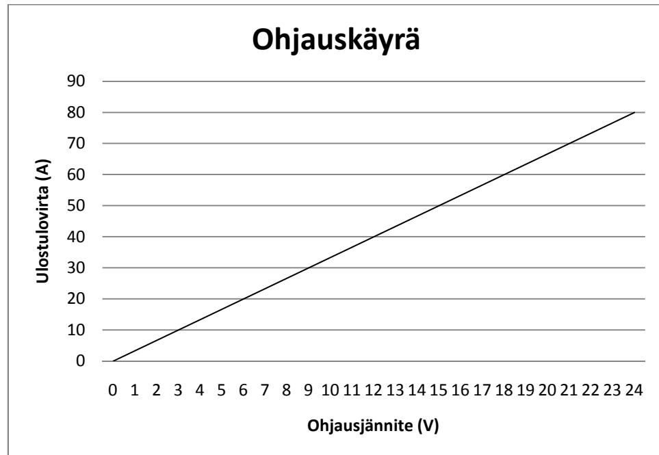
KUVIO 6. Sähkökaapin lähtövirta ohjaukijännitteen funktiona.
