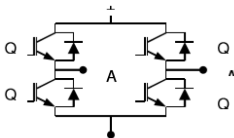
Kuva 12. Suurtaajuuksinen DC/AC-vaihe (NWL DSP PowerPlus Series 6:n tuoteopas 2019).
