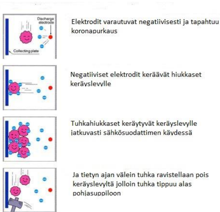
Kuva 4. Sähkösuodattimen tuhkapoiston vaiheet
