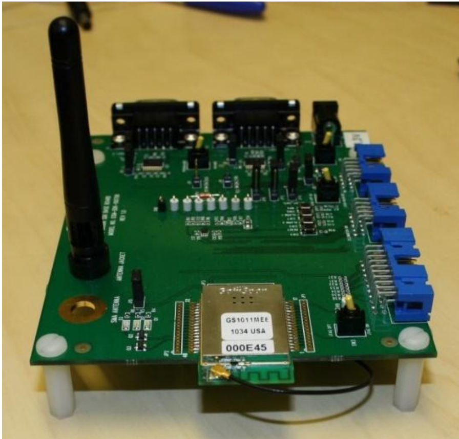
KUVA 10. GainSpan GS1011MEE kehitysalusta
