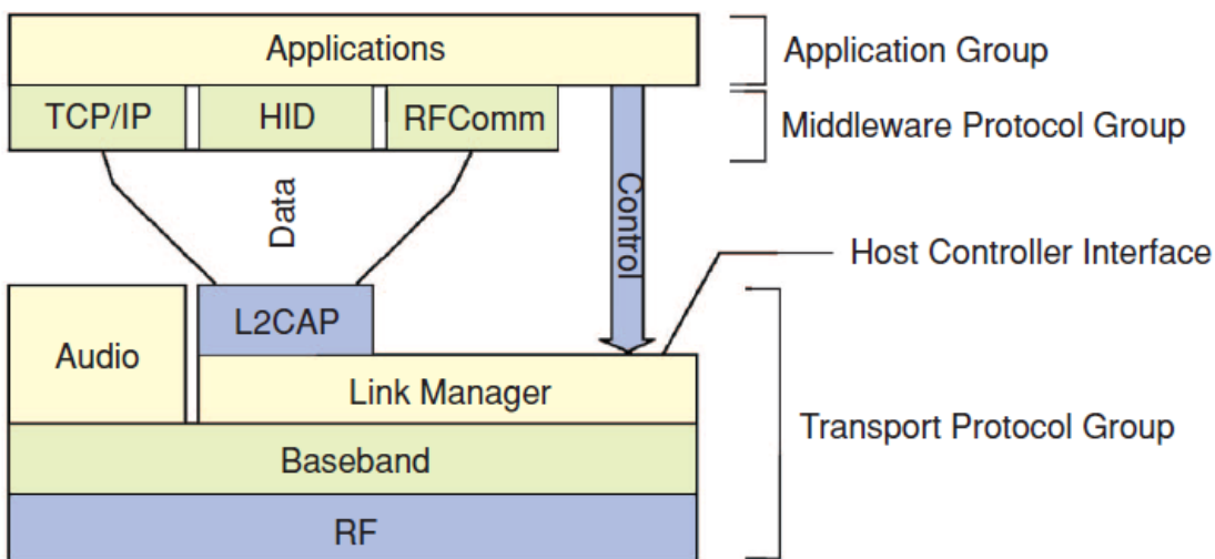
KUVA 3. Bluetoothin protokollapino [11]
