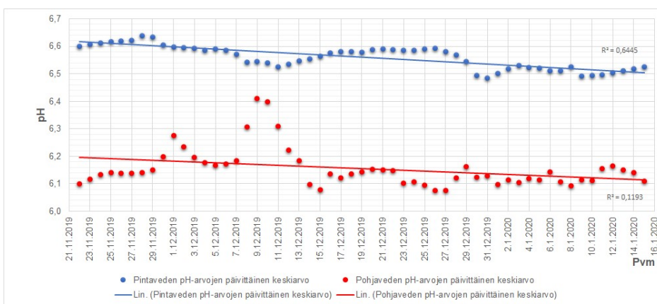
Kuva 3. Pinta- ja pohjavesisondien mitaamat veden pH-arvojen päivittäiset keskiarvot ja regressioviivat.
