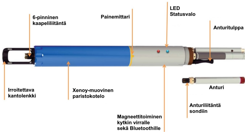
Kuva 1. YSI EXO 1 -vedenlaatusondin havainnekuva (mukaiillen YSI Inc. 2014).
