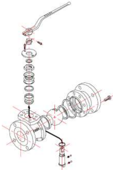
Kuva 7. Palloventtiili /19/
