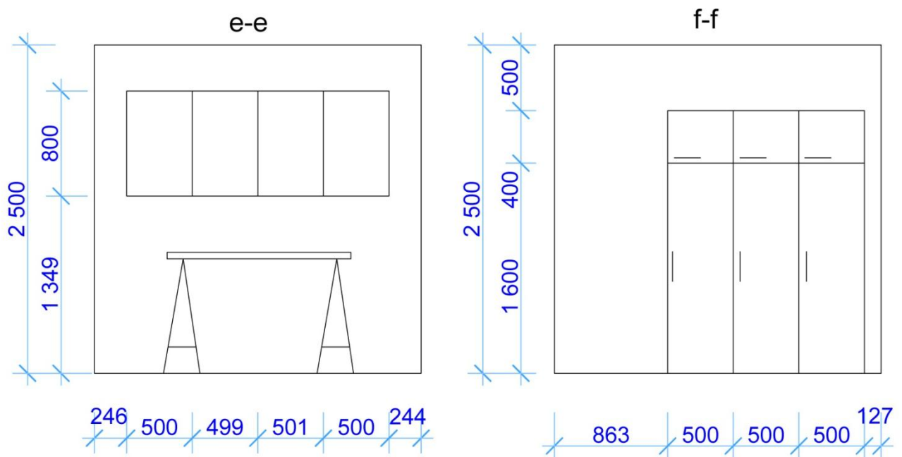
Kuva 44. Suunnitteluhuoneen seinäprojektiot, ei mittakaavassa.
