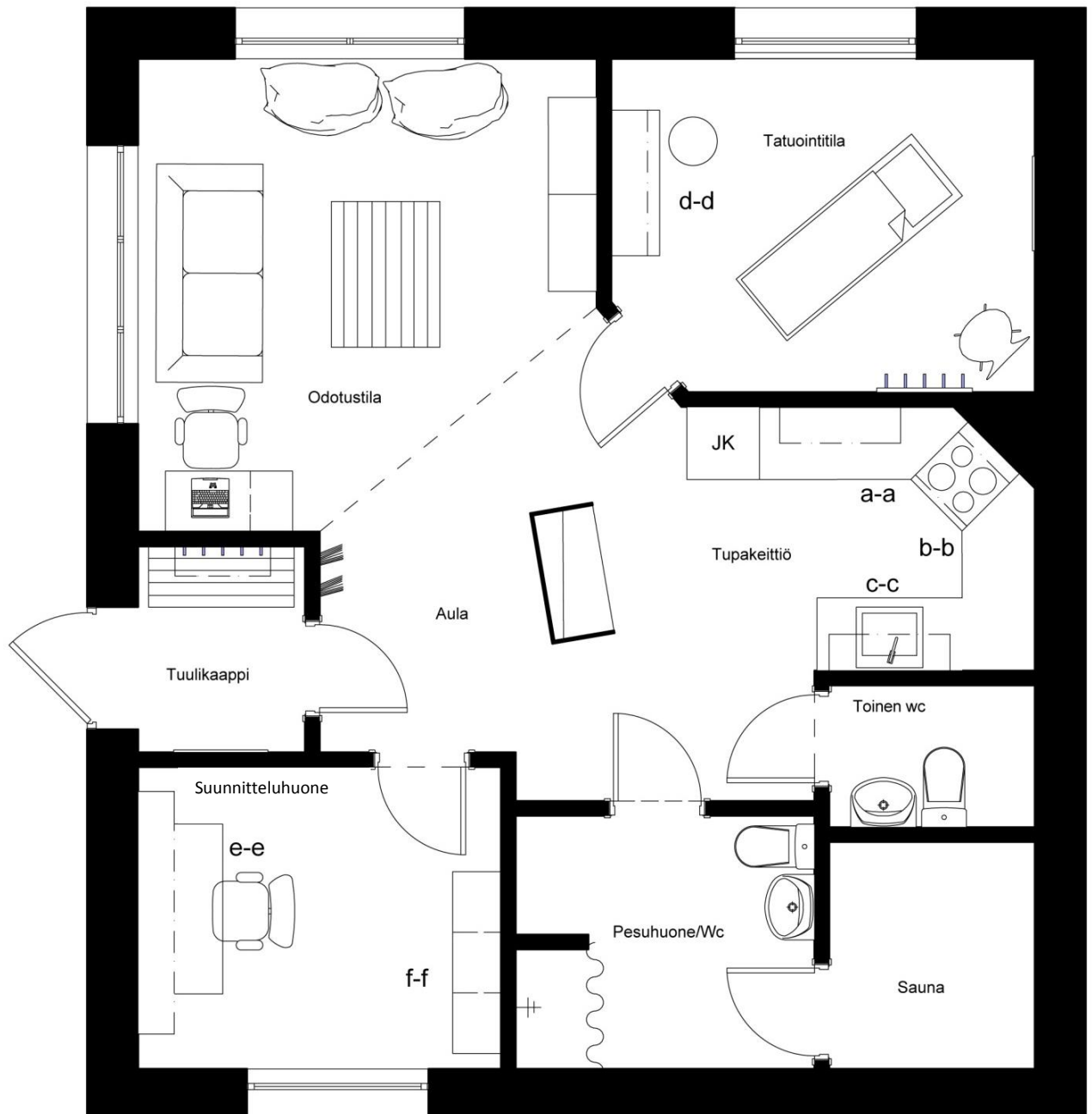
Kuva 27. Pohjapiirros 1:50.
