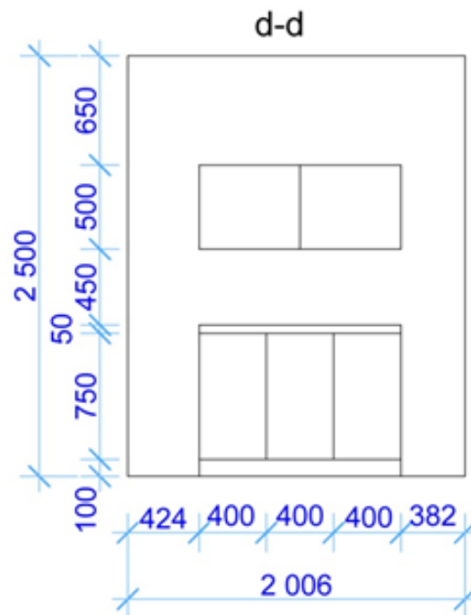
Kuva 43. Tatuointitilan seinäprojektiot, ei mittakaavassa.
