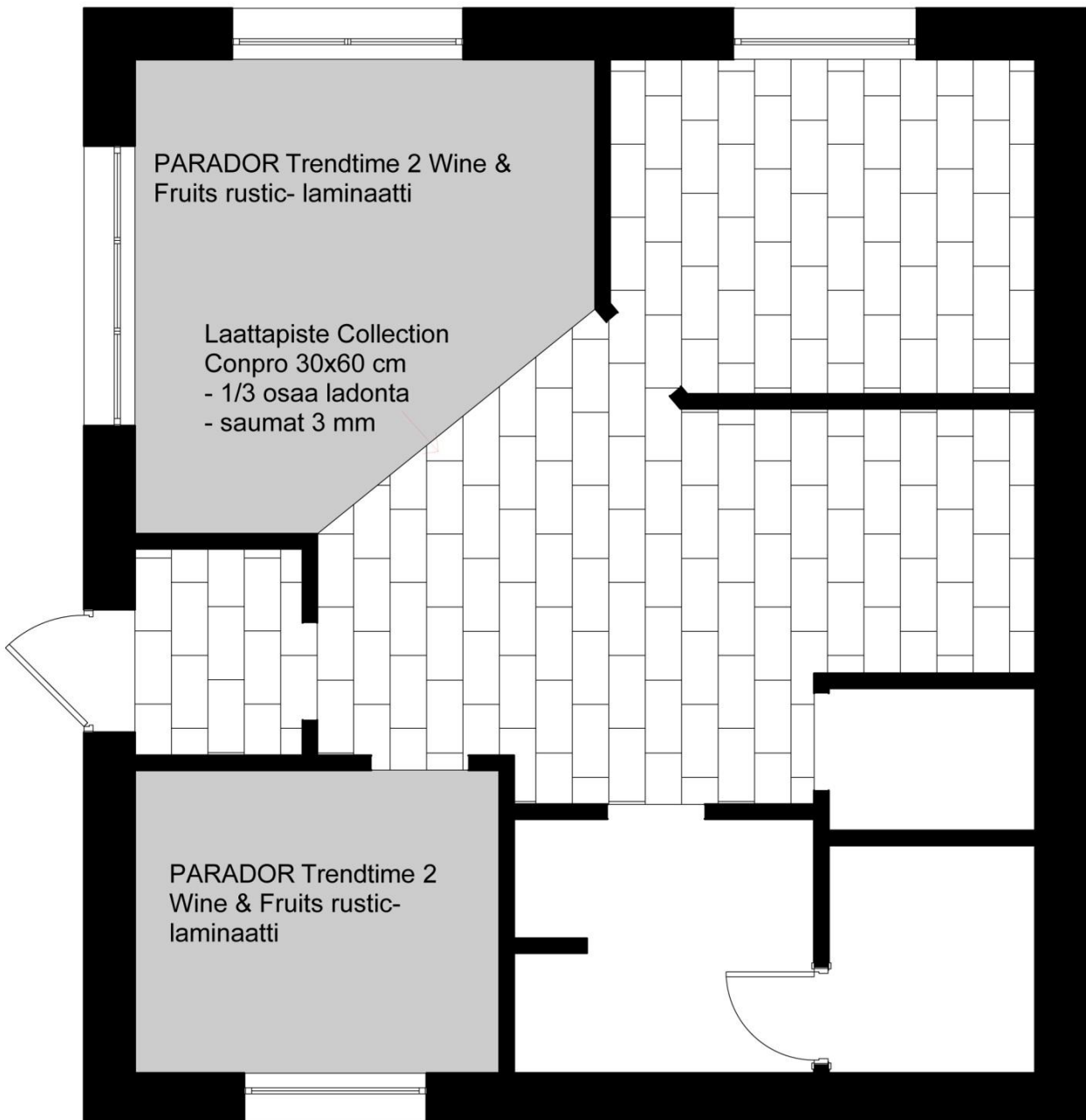
Kuva 30. Lattiapiirros 1:50.
