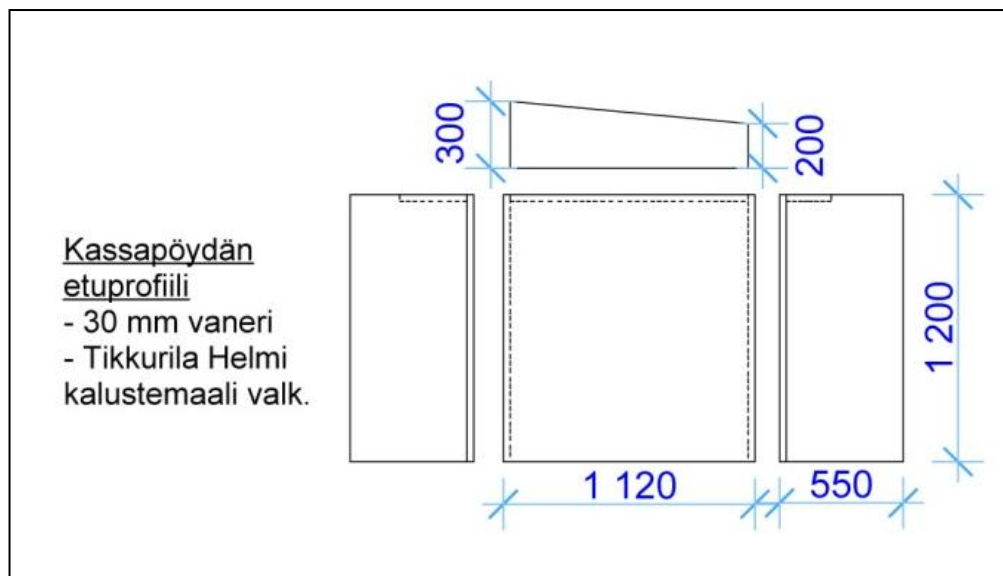
Kuva 57. Kassapöydän peiteprofiili, ei mittakaavassa
