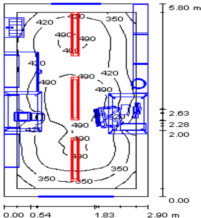
Kuva 20. Toimiston valaistusvoimakkuuskäyrät.
