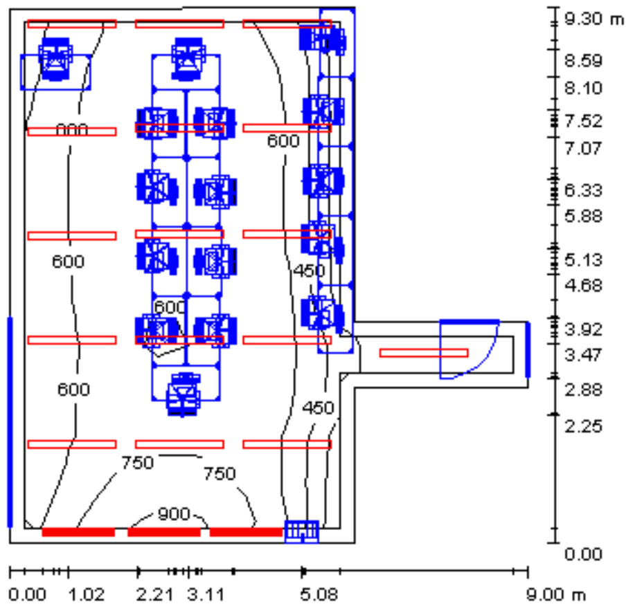
Kuva 17. ATK-luokan valaistusvoimakkuuskäyrät.
