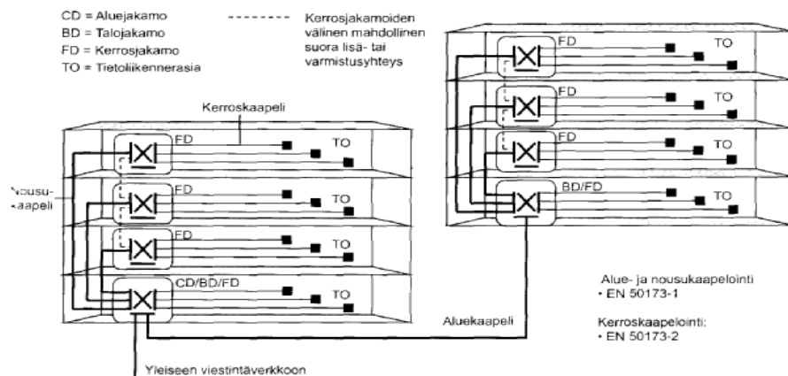
Kuva 9. Toimistokiinteistön yleiskaapelointi esimerkki. /12/
