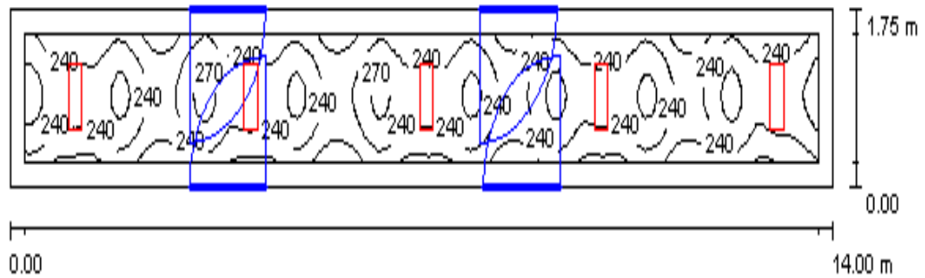
Kuva 23. Käytävän valaistusvoimakkuuskäyrät.
