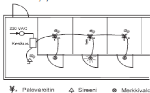
Kuva 11. Palovarotinjärjestelmä. /9/
