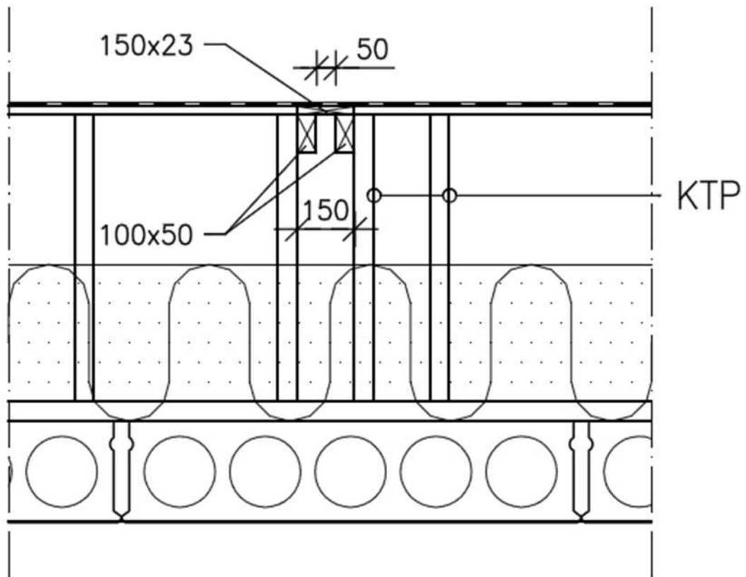
Kuva 8 Vesikattoelementtien välinen liitos
