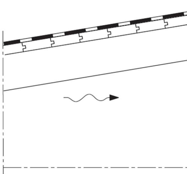
Bitumikermikate rakennuselostuksen mukaan Raakaponttilaudoitus rakennesuunnitelman mukaan Kattokannattajat ja tuulettuva ilmatila (vähintään 100 mm) rakennesuunnitelman mukaan
