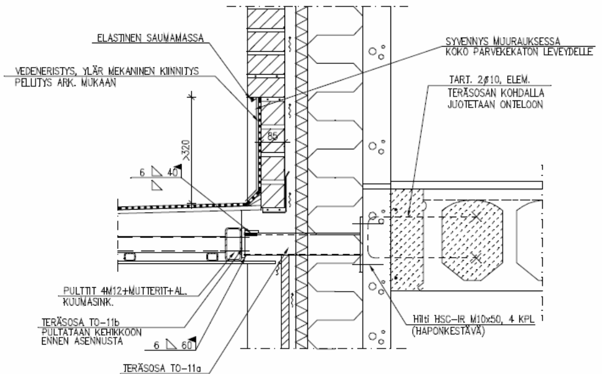
Kuva 11. Teräsbetoni-laatan liittymädetalji runkoon. [3.]
