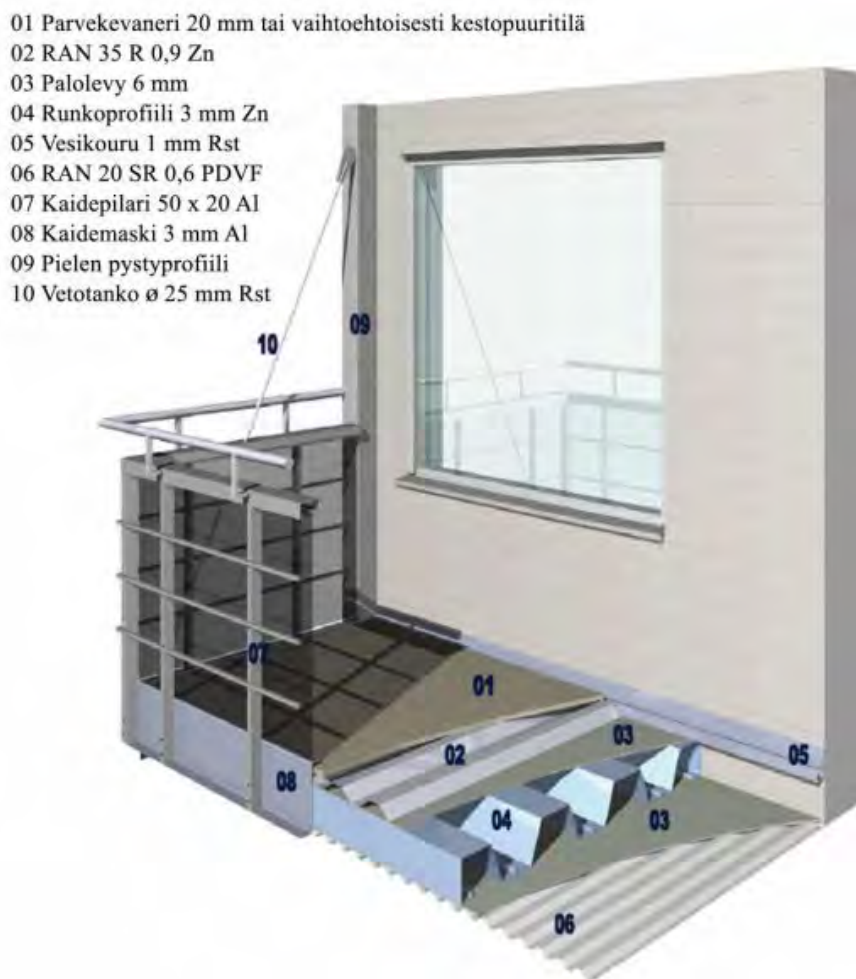
Kuva 27. Havainnekuva teräsparvekkeesta, KT-Tähtinen. [34.]
