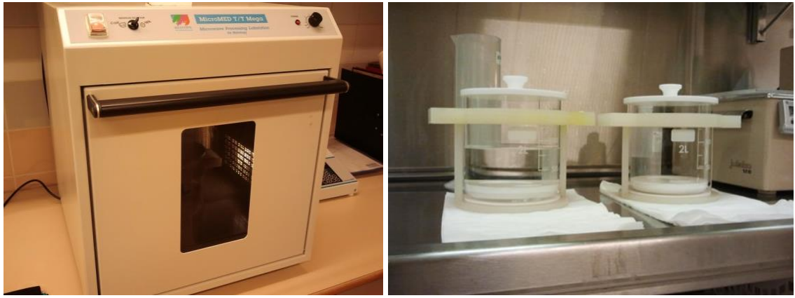
KUVA 11. Esikäsitellyissä käytetty MikroMed T/T Mega -laite ja esikäsitteilymaljat (Kuva: Elina Virkkunen 2012)
