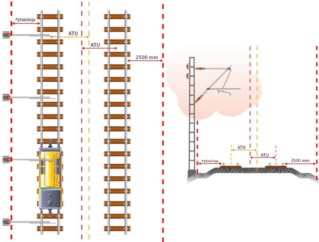
Kuva 7. Ratatyön suojalottuma [8, liite1]
