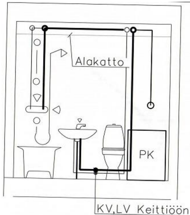
Kuva 7. Vesijohdot alakatosta vesikalusteisiin ja seinän läpi keittiöön (RIL 252-2-2009, 14)
