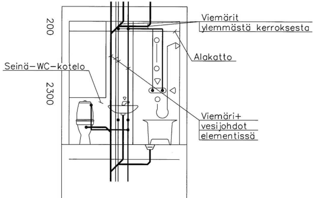
Kuva 8. Viemärivetojen ratkaisuvaihtoehto (RIL 252-2-2009, 18)
