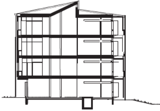
Kuvio 2. Paikallavaaletun kerrostalon runkorakenne.
