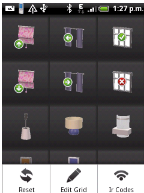
Kuva 2. Housemate-ohjelman käyttöliittymä
