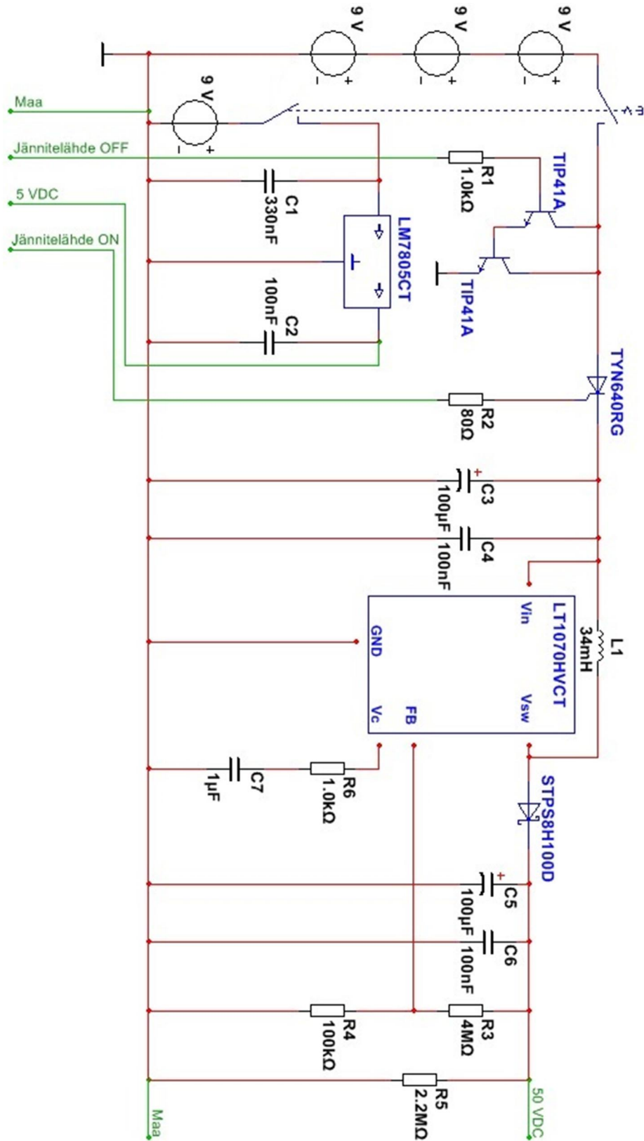
LIITE 1. Jännitelähteen kytkentäkaavio
