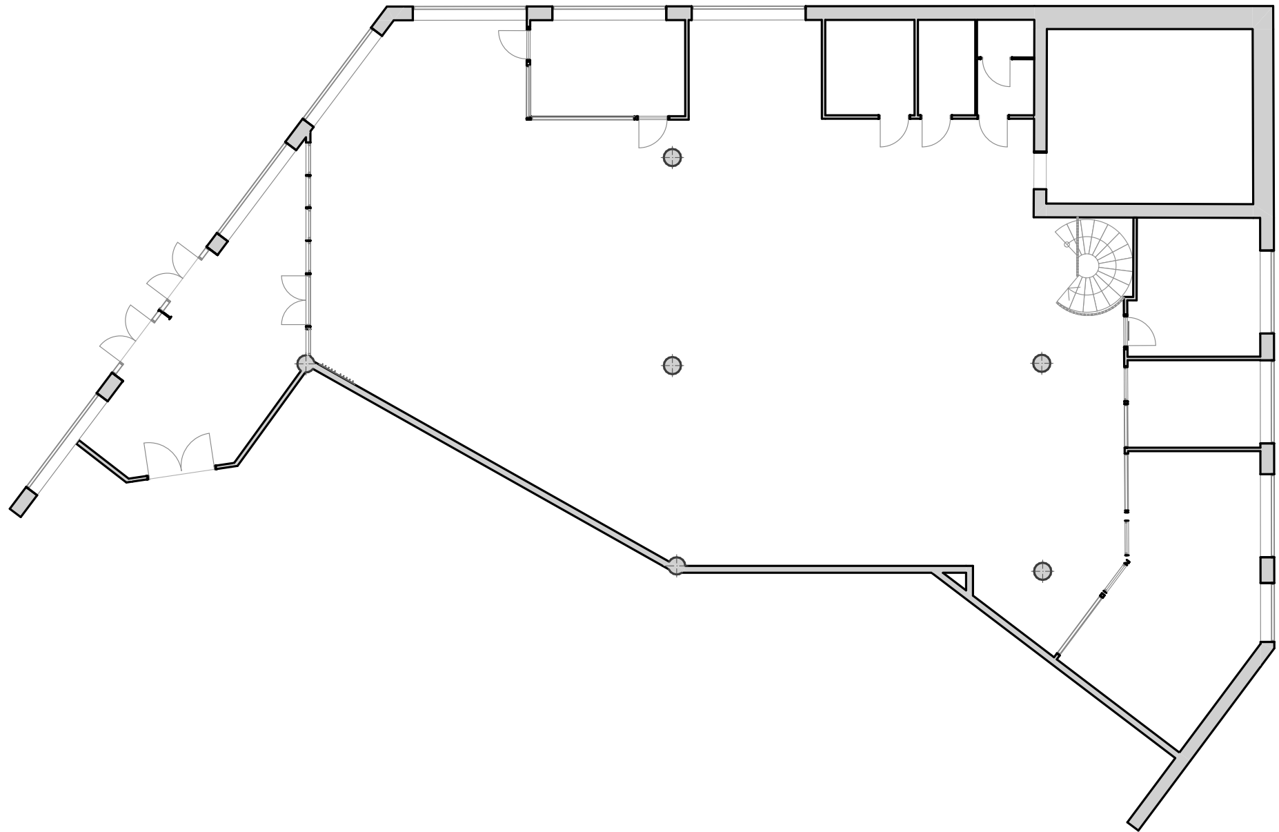
Kuva 17. Alkuperäinen pohja puhtaaksi piirrettynä
