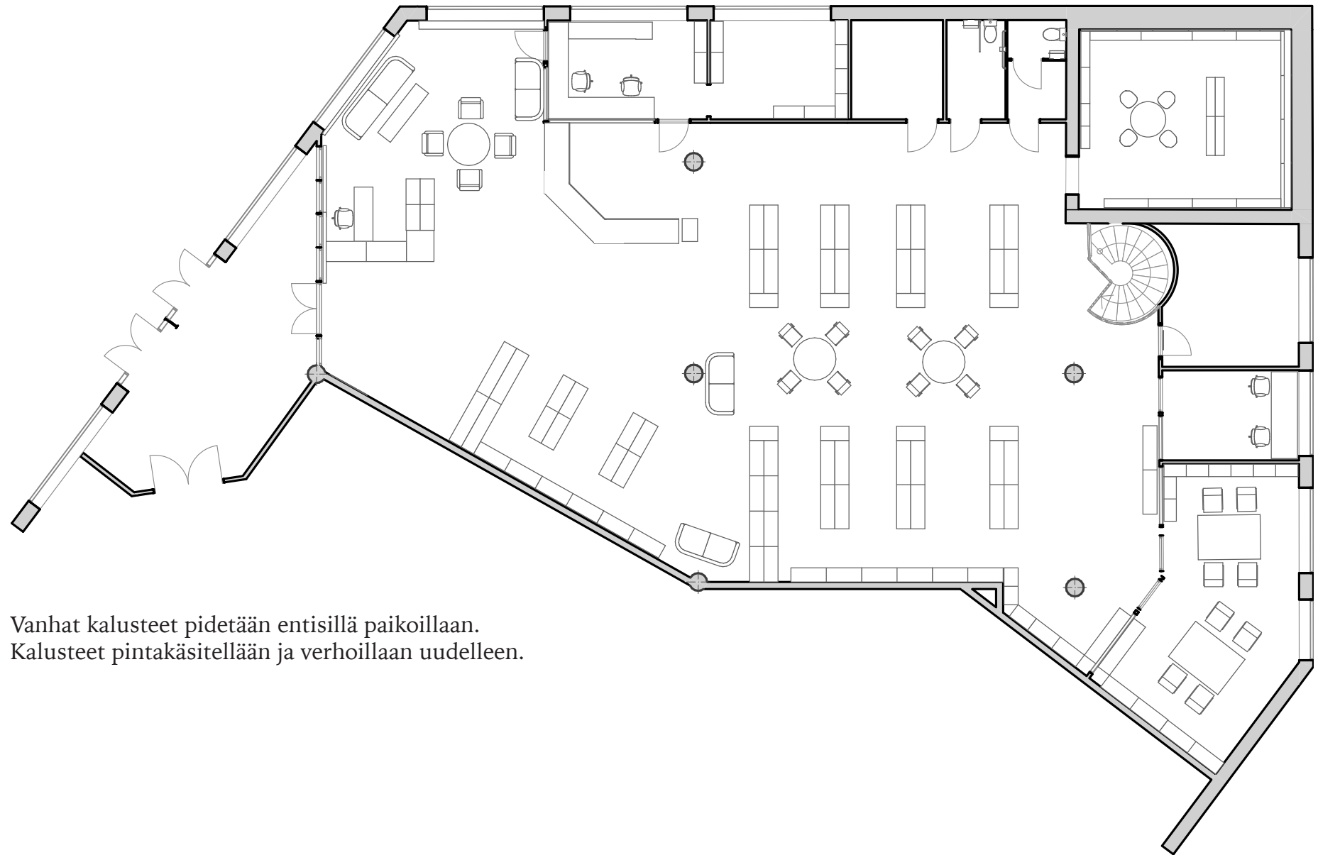
Kuva 19. Pohjakuva kalusteilla
