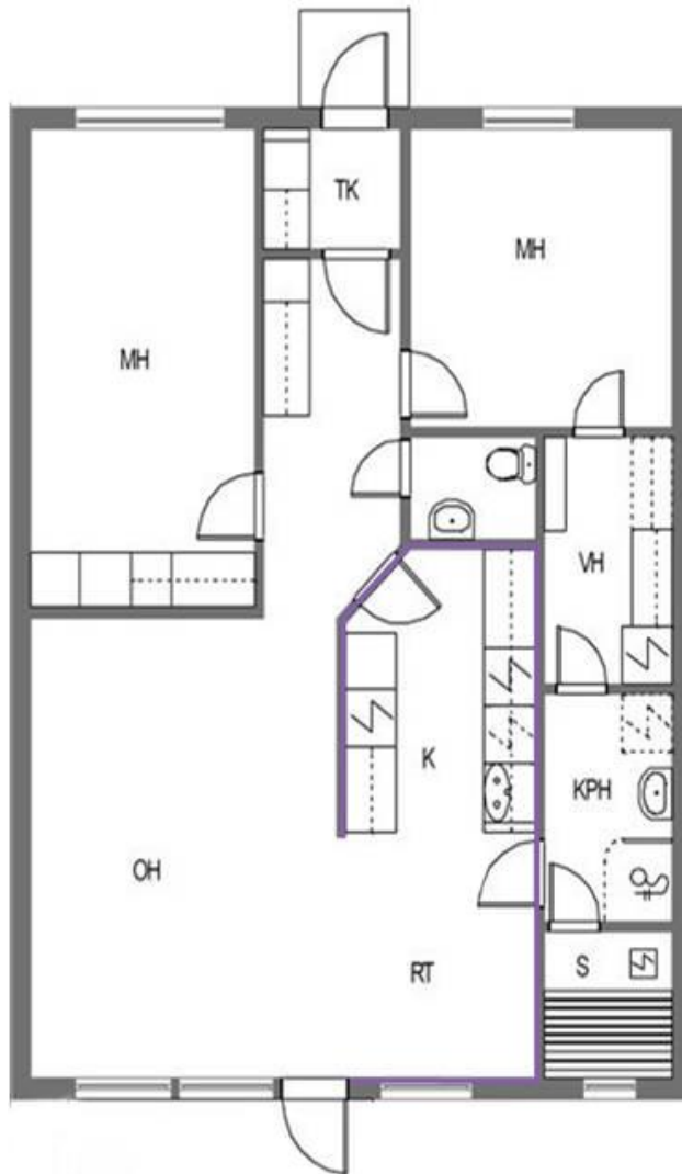
Kuva 4. Asunnon pohjakuva, ei mittakaavassa.
