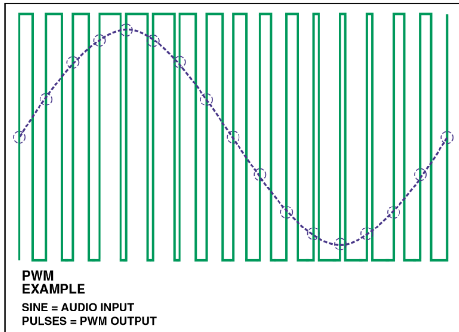
Kuva 4. PWM-esimerkki. [2]
