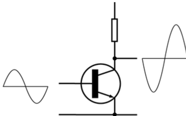
Kuva 1. A-luokan vahvistin. [1]
