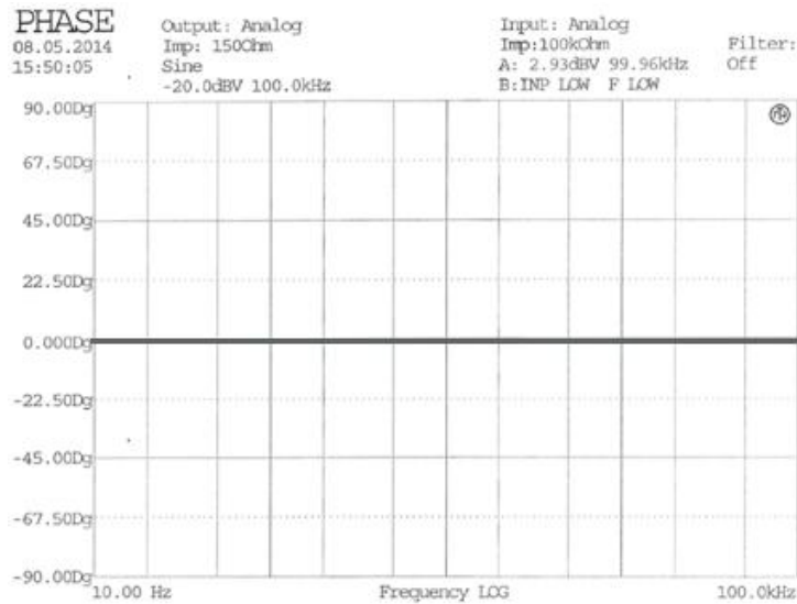
Kuva 24. Vahvistimen vaihevaste.
