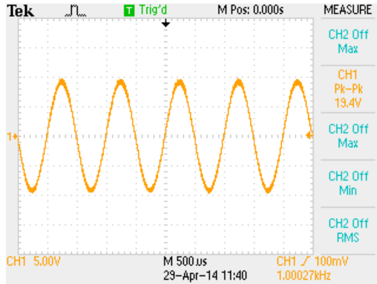
Kuva 19. Toinen transient-mittaustulos.
