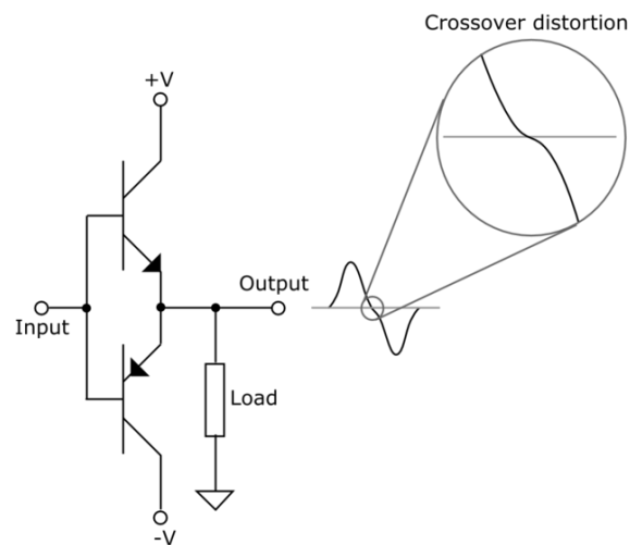
Kuva 2. B-luokan vahvistimen ylimenosärö. [3]
