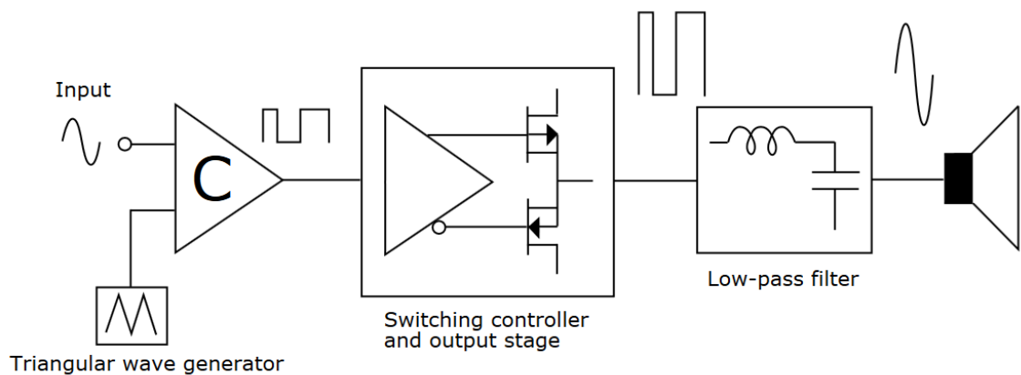
Kuva 3. D-luokan vahvistimen lohkokkaavio. [1]
