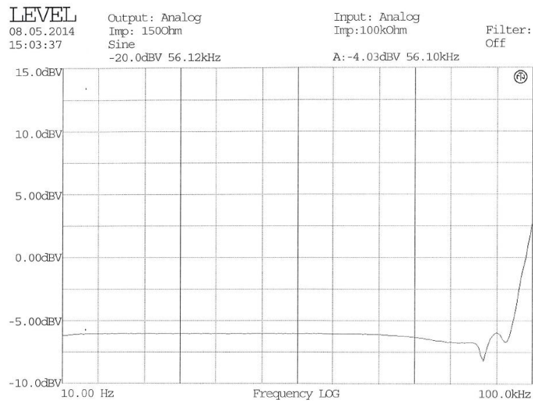
Kuva 23. Vahvistimen amplitudivaste.
