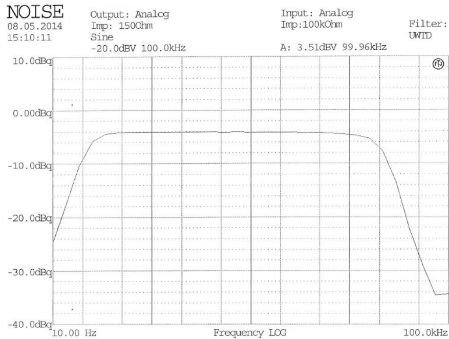
Kuva 22. Kohinamittaus.
