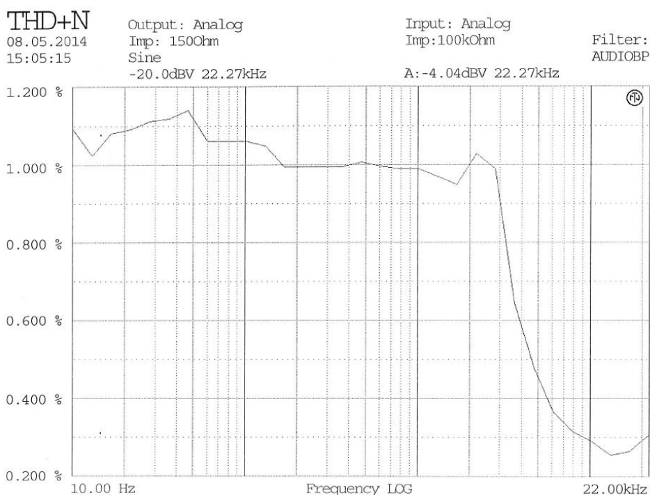
Kuva 21. THD+N -mittaus.
