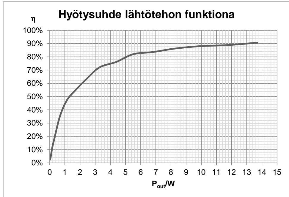
Kuva 25. Hyötysuhde lähtötehon funktiona
