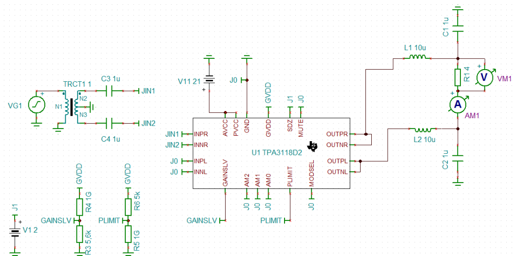
Kuva 11. TPA3118D2-kytkentä TINA-TI-ohjelmassa.
