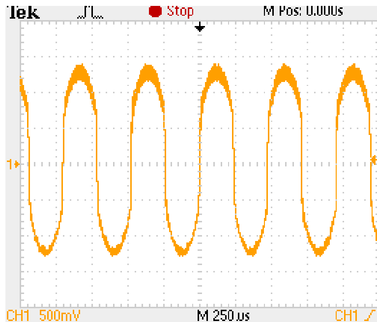
Kuva 18. Ensimmäinen transient-mittaustulos.
