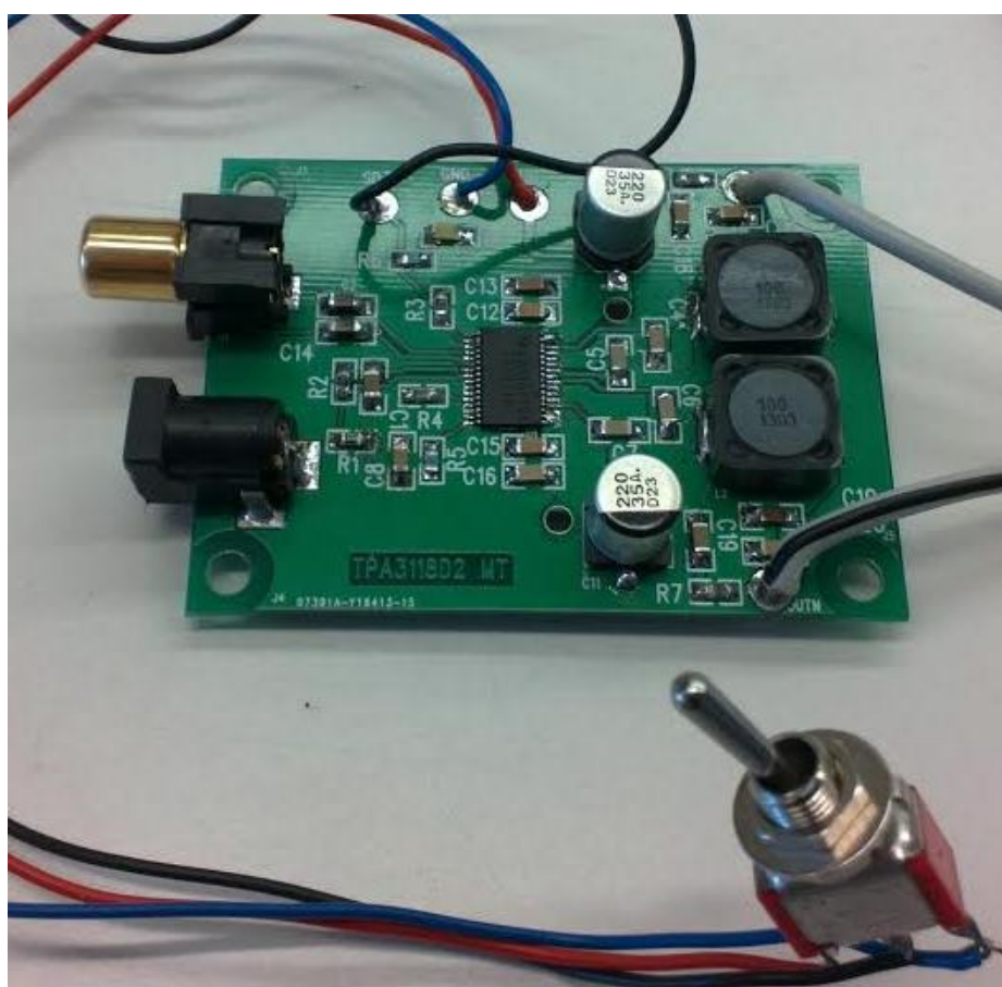
Kuva 17. Valmis piirilevy.
