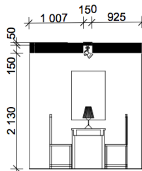
Leikkaus D-D
