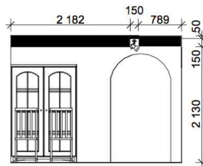
Leikkaus B-B
