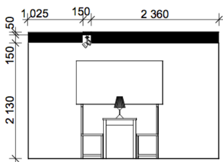
Leikkaus A-A
