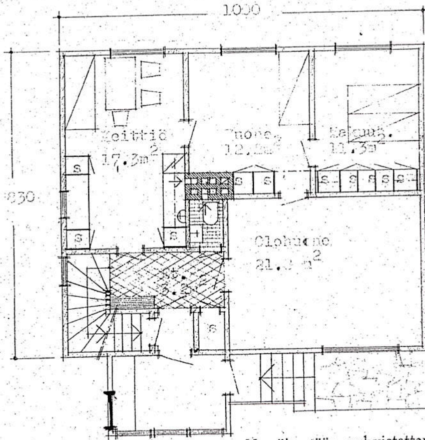
Asuinkerros
