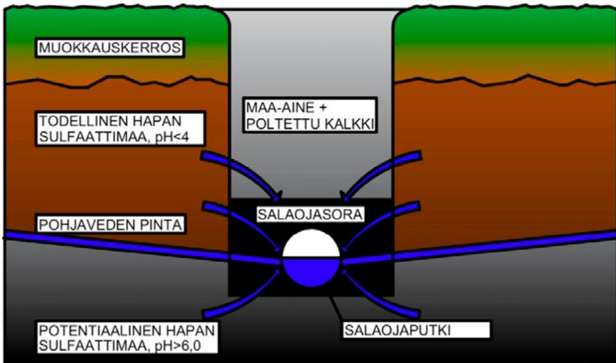
Kalkkisuodinojan periaatekuva. Kuva: Markus Mononen, mukailen MMM 2009.
