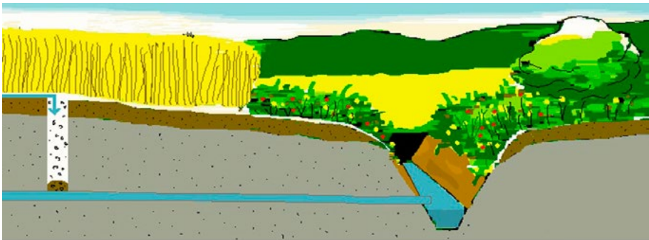
Pintavesien ohjaaminen rinnepellolta kalkkisuodinojaan vähentää vesistöjen fosforikuormitusta.
