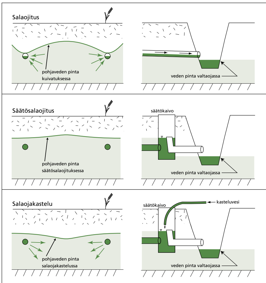
Salaojituksen, säätösalaojituksen ja säätekastelun periaatteet sekä pohjaveden pinta maaperässä. Kuva: Salaojayhdistys ry.
