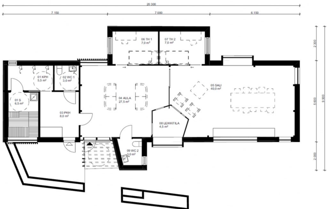
KUVA 1. Pohjapiirustus (kuva: Jenni Myllynen, 2023).
