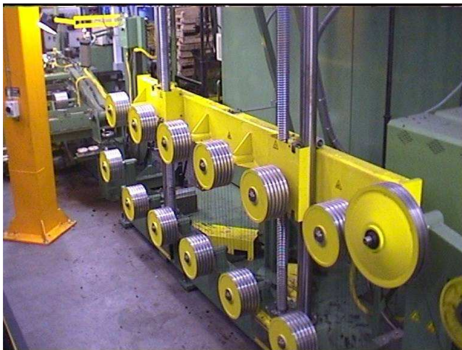
Kuva 6 Langan jäähdytysreservi /5/
