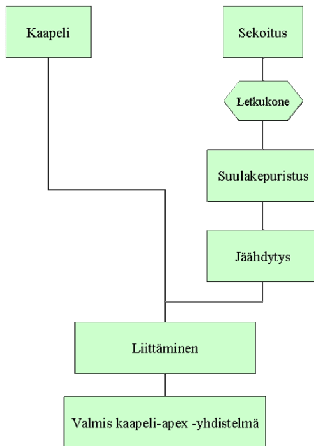
Kuva 10 Kaapelin liuskausprosessi /5/
