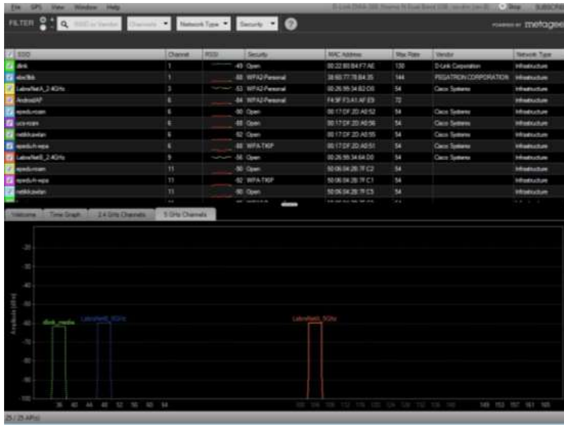
Kuvio 23. inSSIDer 5 GHz:n taajuus.
