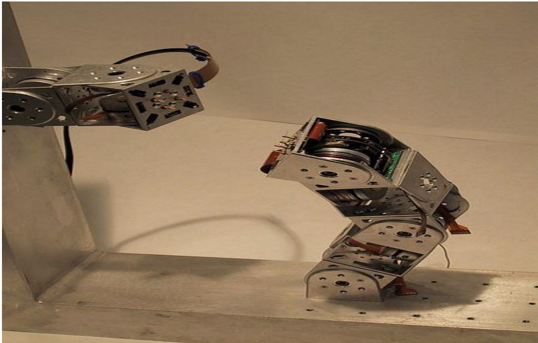
Kuva 8. PolyBot 3G -Robotti. (wikimedia.org)
