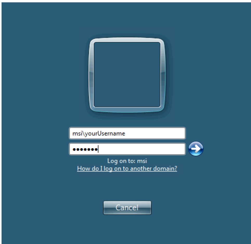
Kuva 2. Kirjautumisikkuna.
