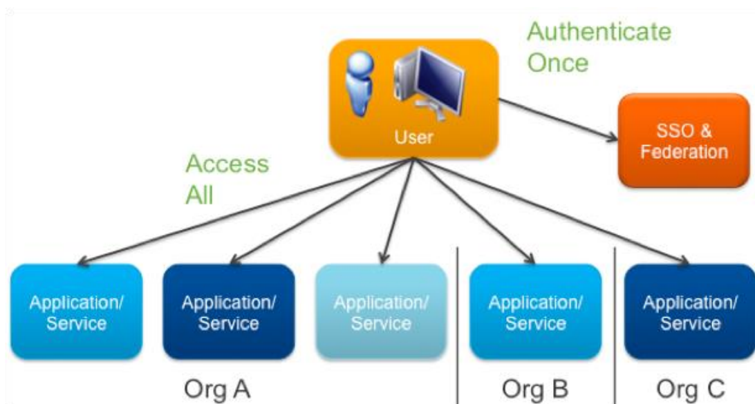
Kuva 5. Kertakirjautuminen.
