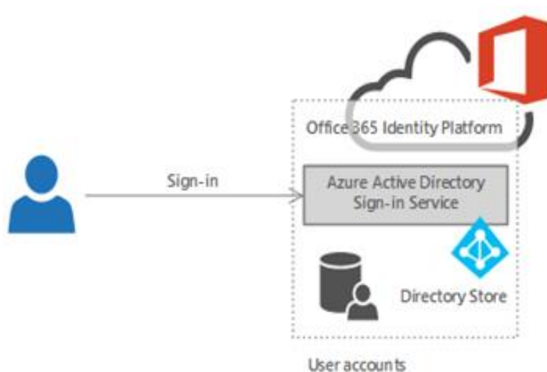
Kuva 11. Pilvi-identiteetin malli.
